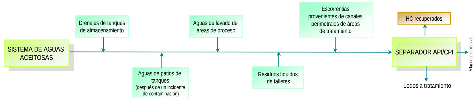
Figura 7.16 Descargas a sistemas de aguas aceitosas y separador API/CPI
