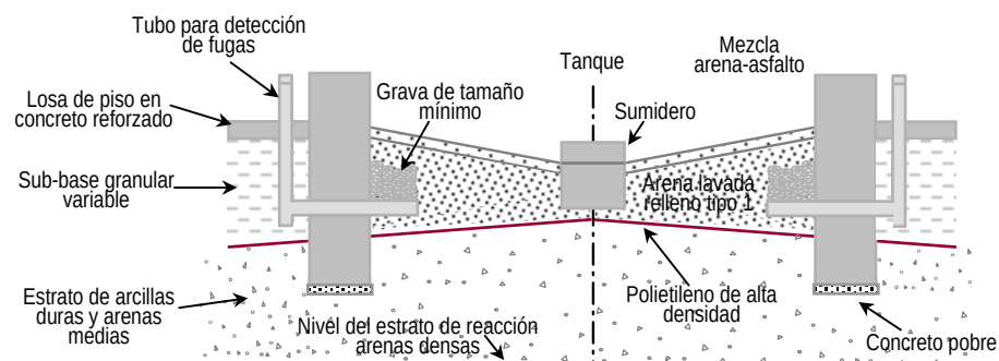
Corte A-A
