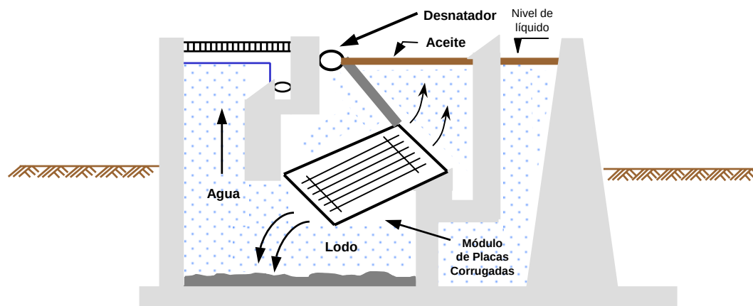
Figura 5.10 Esquema del Separador CPI
