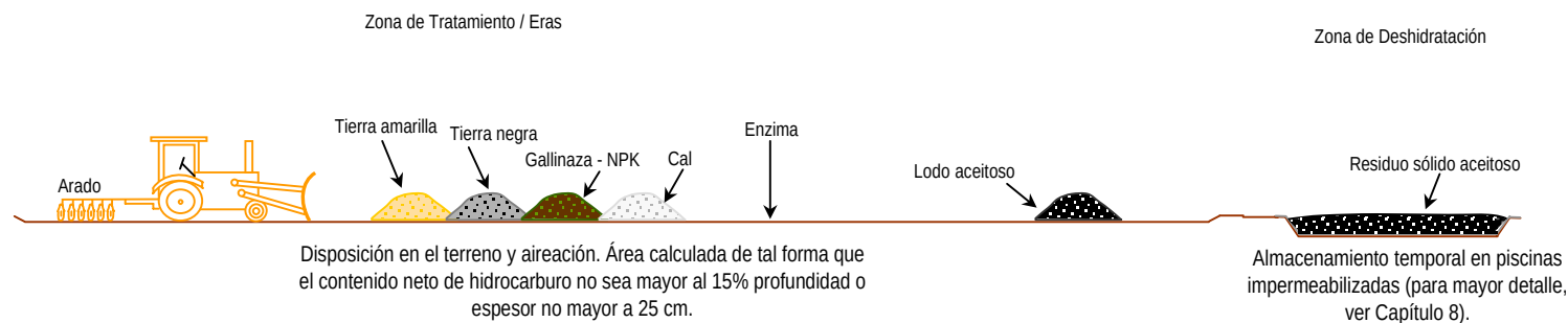
Figura 5.11 Esquema de Tratamiento de Residuos Aceitosos
