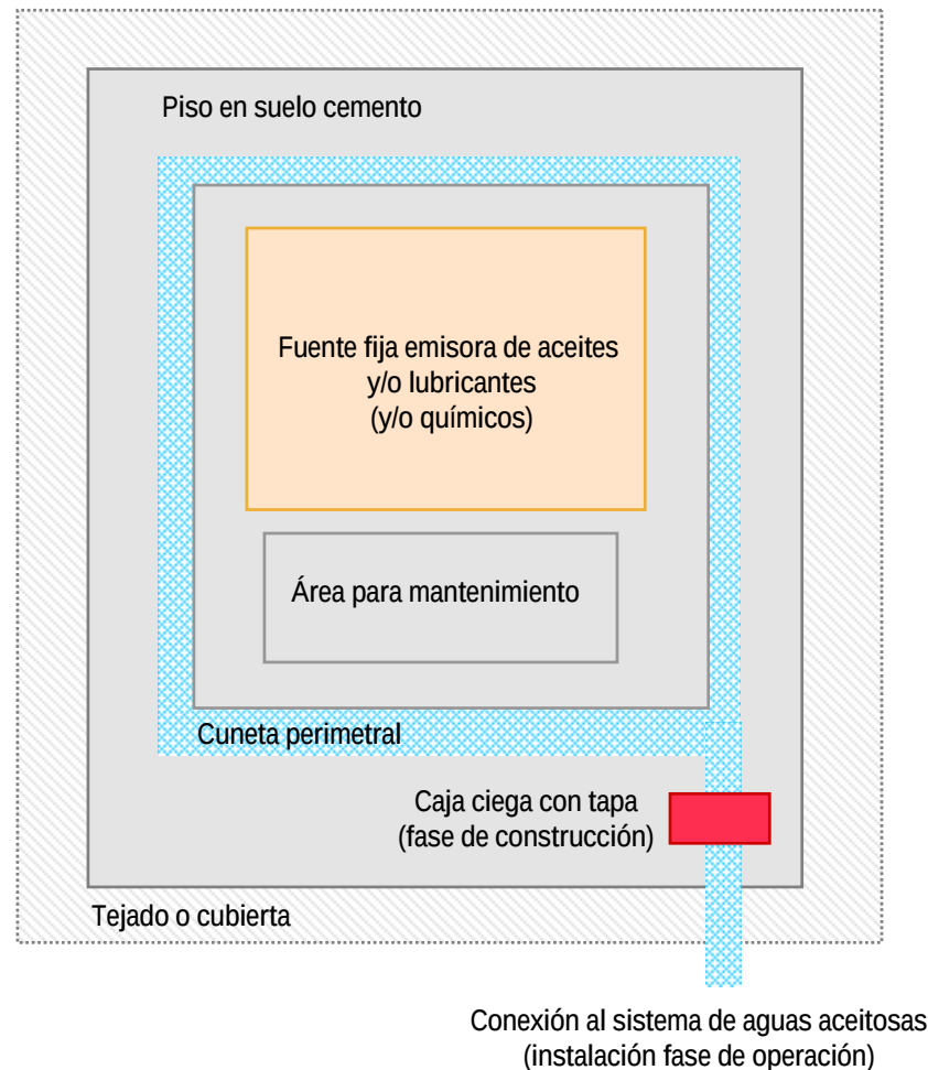
Figura 7.8 Manejo de Grasas y Lubricantes en Edificaciones (vista en planta)
