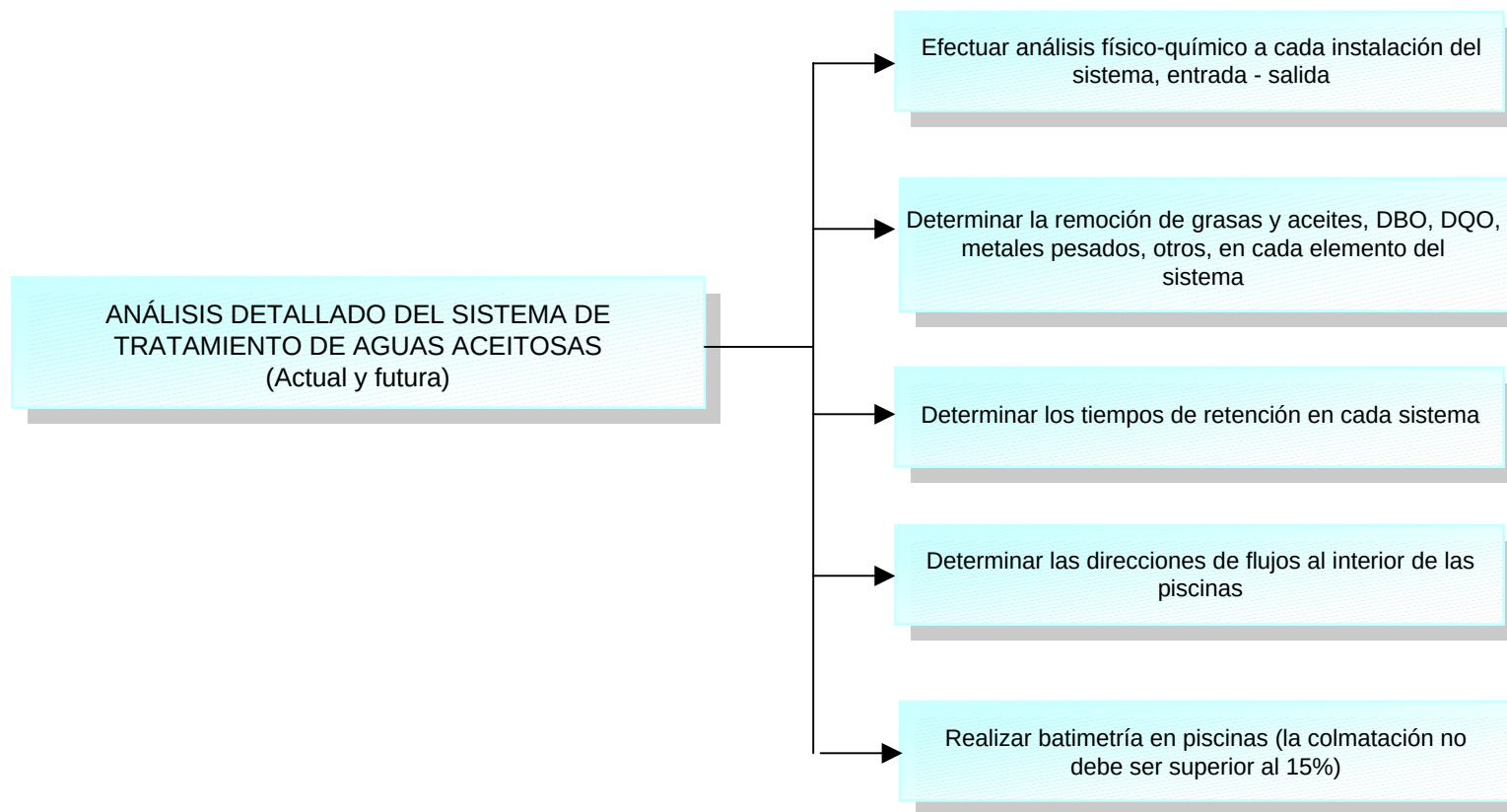
Figura 9.1 Esquema para el diagnóstico del sistema de tratamiento de aguas
