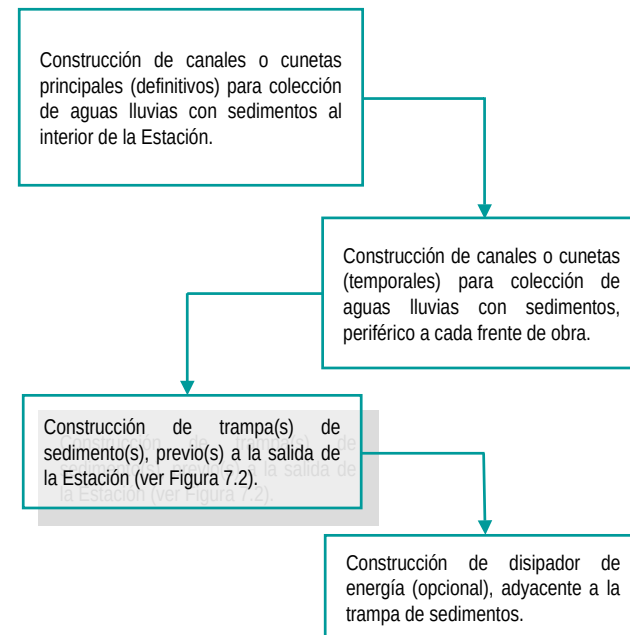
Figura 7.5 Manejo de Aguas con Sedimentos
